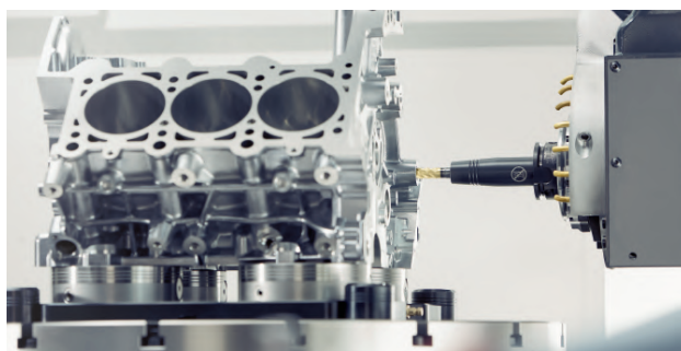
TENDO Slim 4axによるシリンダーヘッド加工
